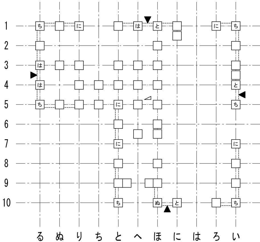
1階柱壁伏図
