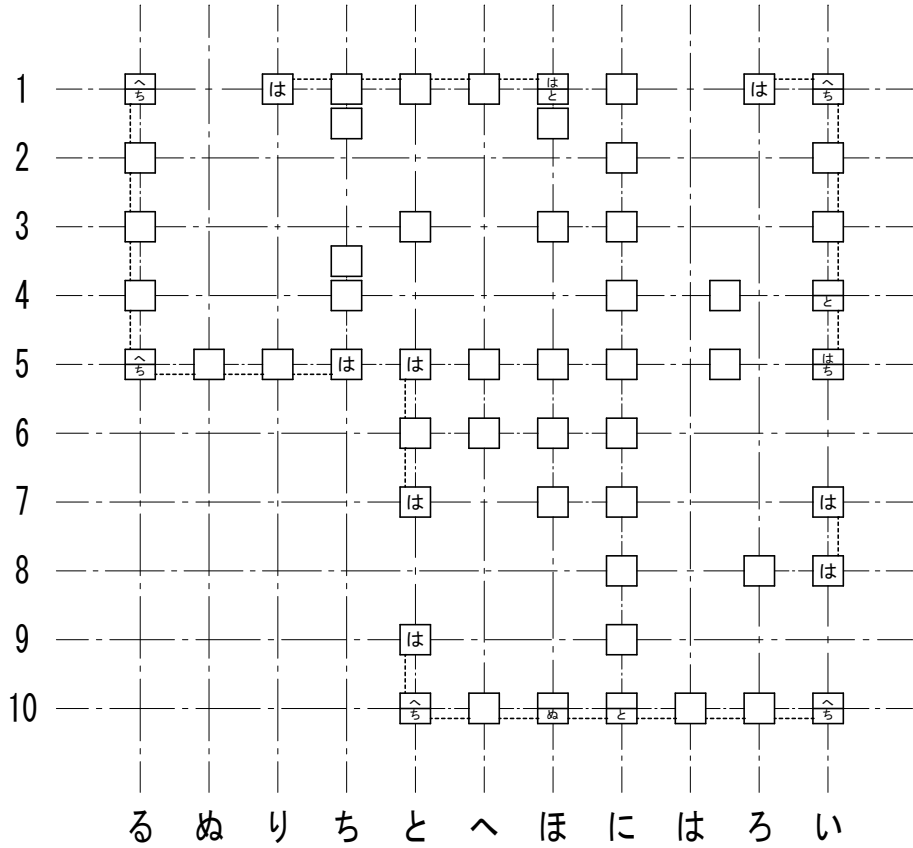
2階柱壁伏図
